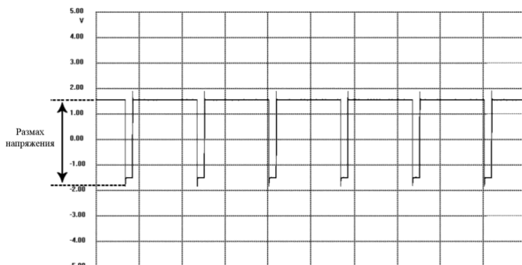
Рисунок 19-2. Пример сигнала прямоугольной формы
